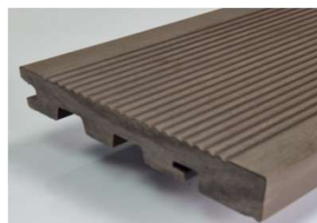
Edge Board
